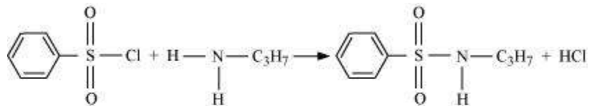
Benzenesulphonyl chloride
