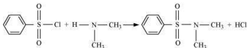
Benzenesulphonyl chloride
